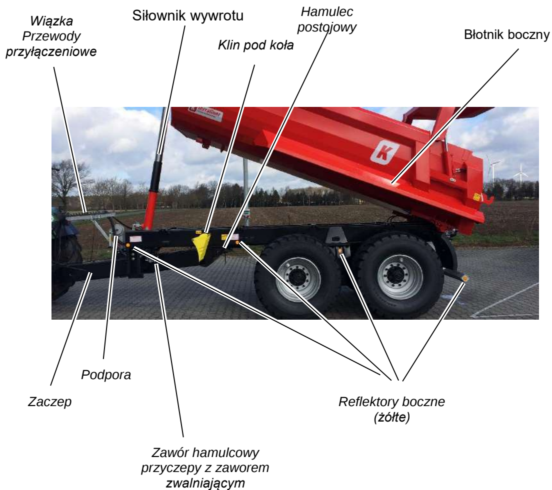
Ilustracja 12: Rama modelu MUP 20 HP, widok z przodu z lewej strony
