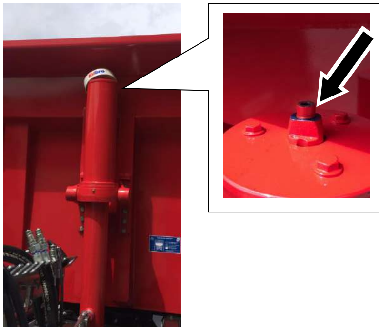
Ilustracja 41: Odpowietrzanie siłownika wywrotu
