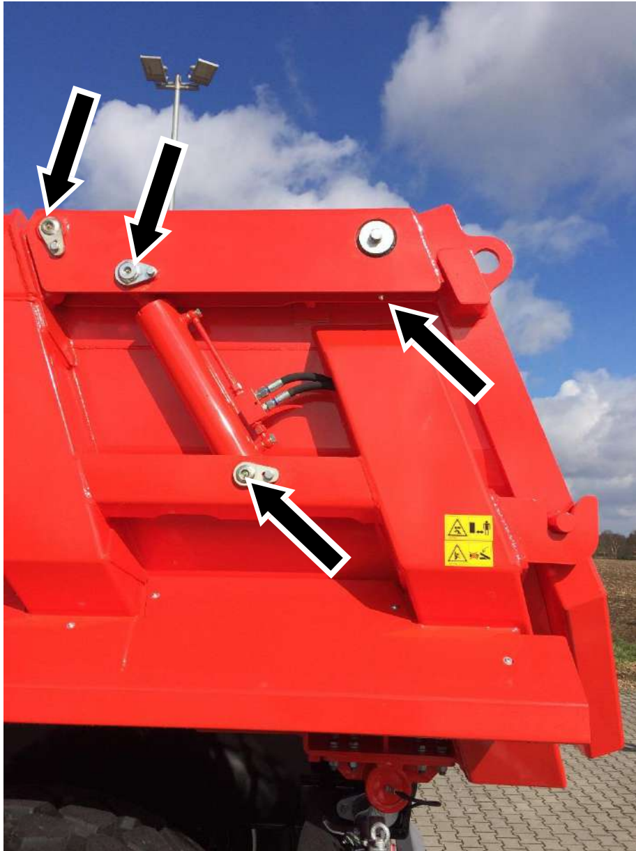
Ilustracja 46: Smarowanie klapy tylnej
