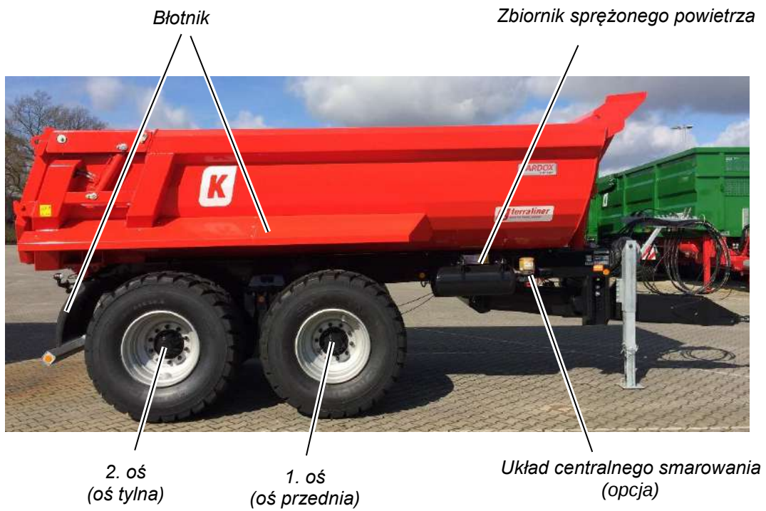
Ilustracja 14: MUP 20 HP, widok z prawej strony
