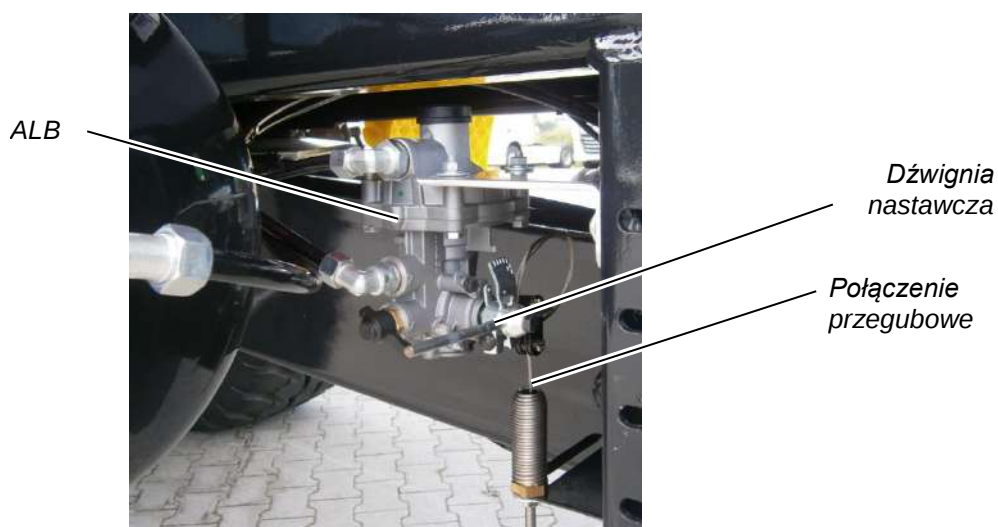
Ilustracja 20: ALB, tutaj: MUP 20 HP
