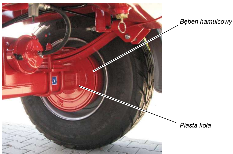
Ilustracja 38: Bęben hamulcowy i piasta koła
