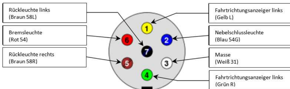
Ilustracja 58: Wtyczka 7-pinowa
