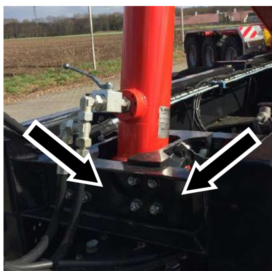
Ilustracja 47: Łożyska wywrotu i siłownik wywrotu
