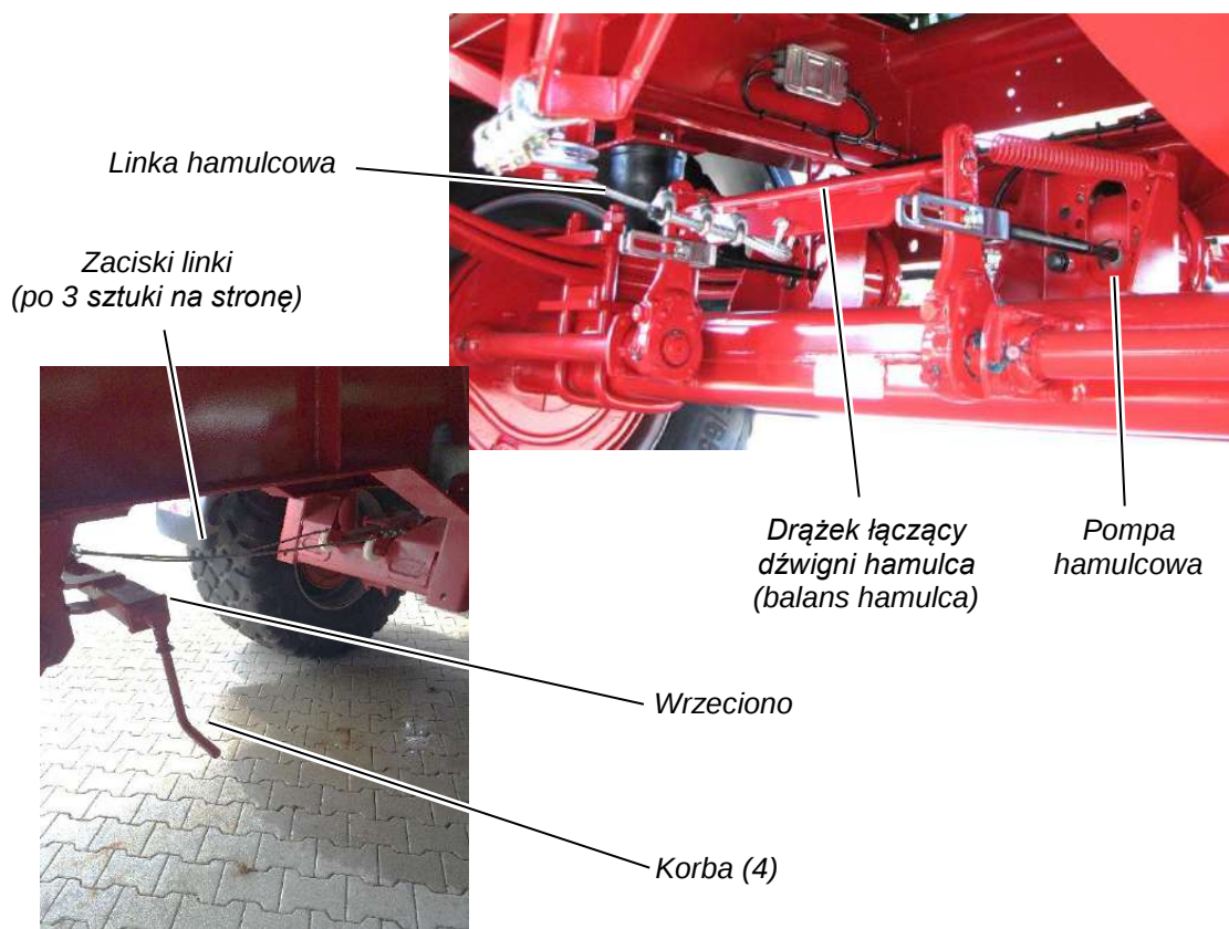
Ilustracja 56: Hamulec postojowy tylnej osi
